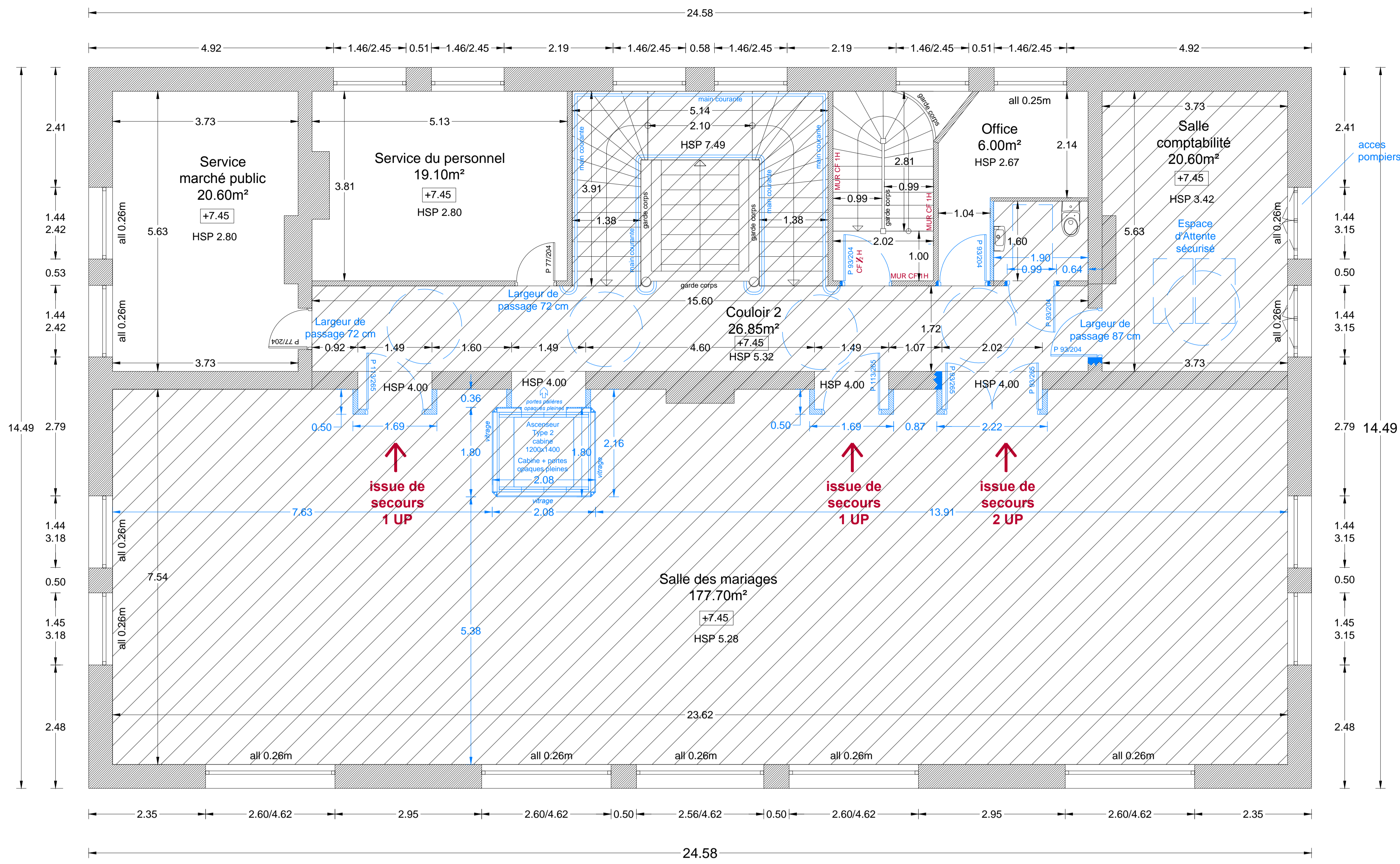
PLAN R+2 ECH : 1/50
