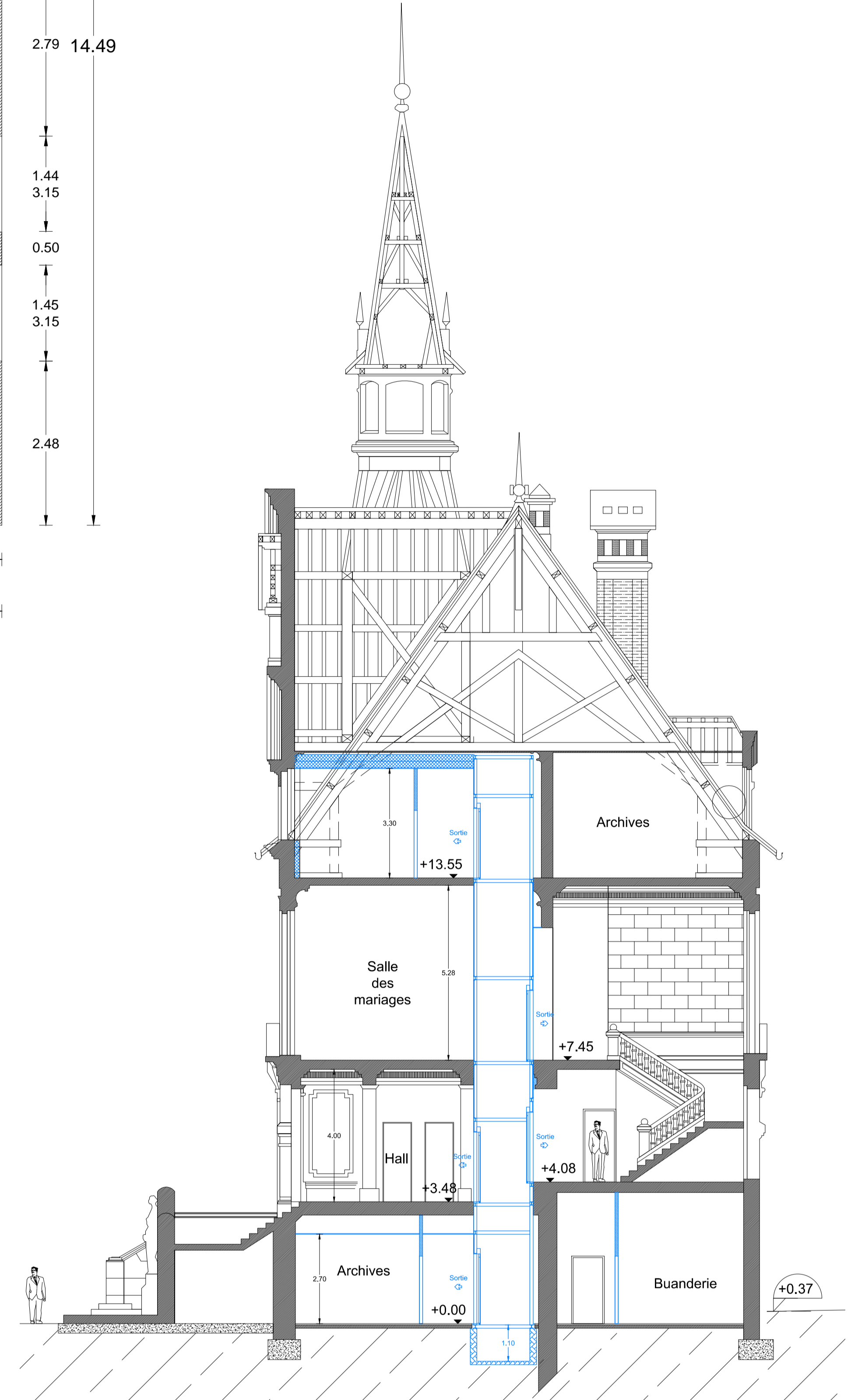
COUPE SUR ASCENSEUR ECH : 1/100
