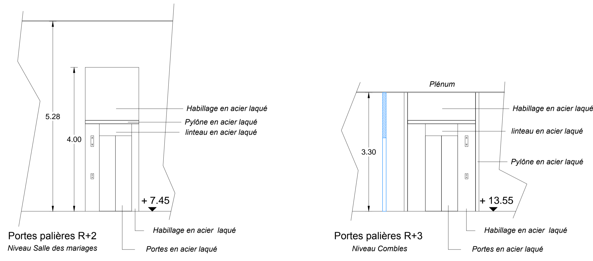
ELEVATIONS PORTES PALIERES ASCENSEUR ECH : 1/50
