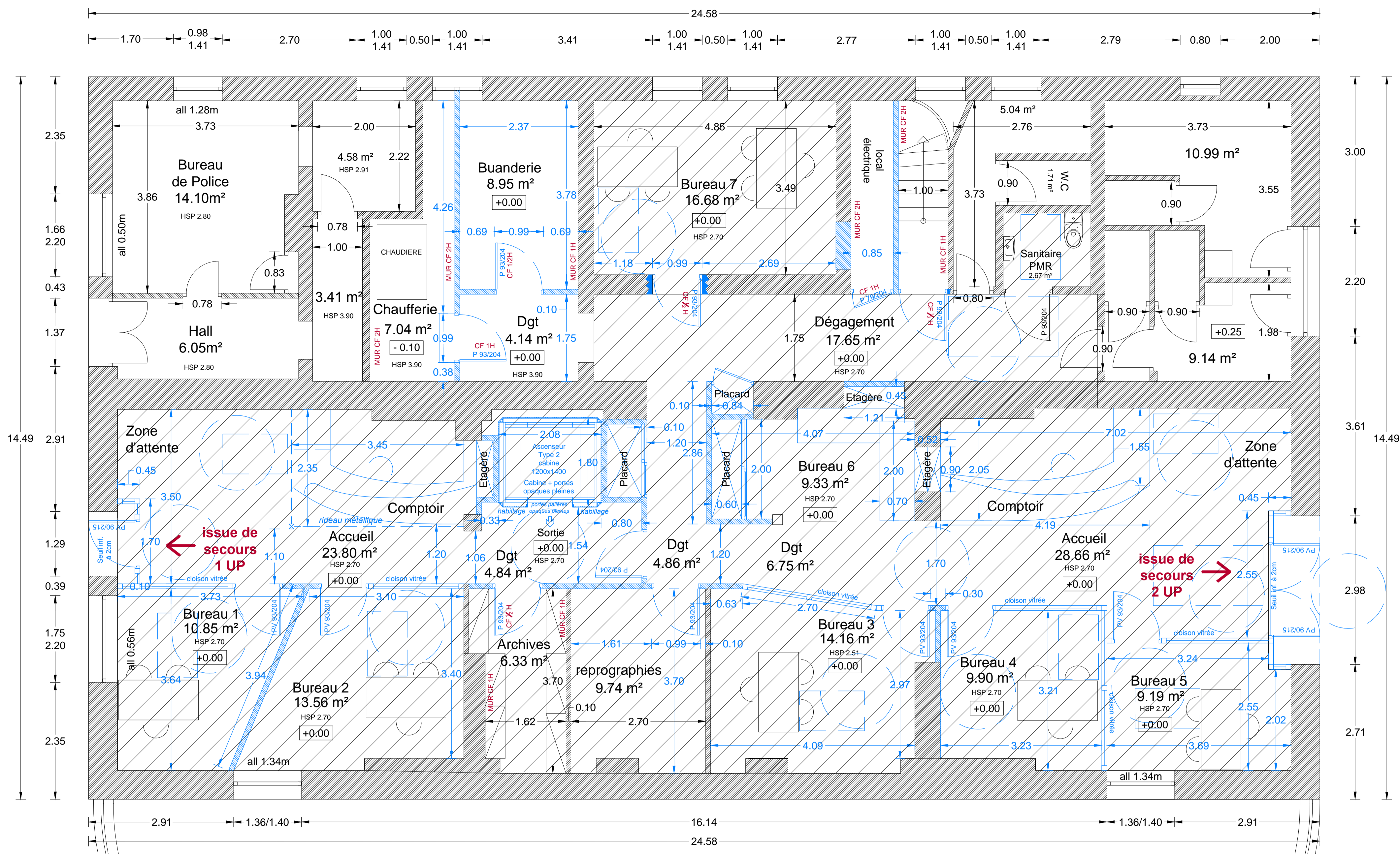
PLAN RDC ECH : 1/50
