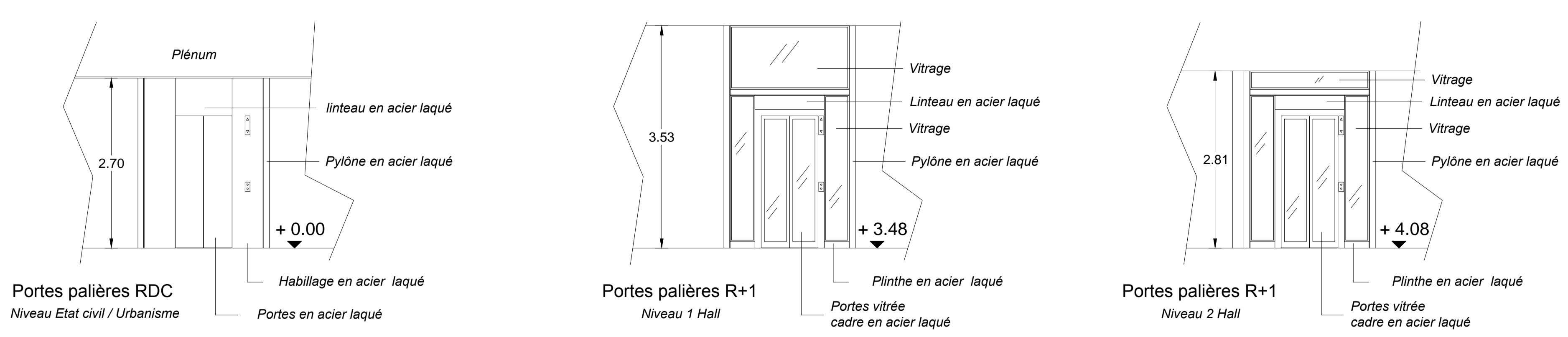
ELEVATIONS PORTES PALIERES ASCENSEUR ECH : 1/50
