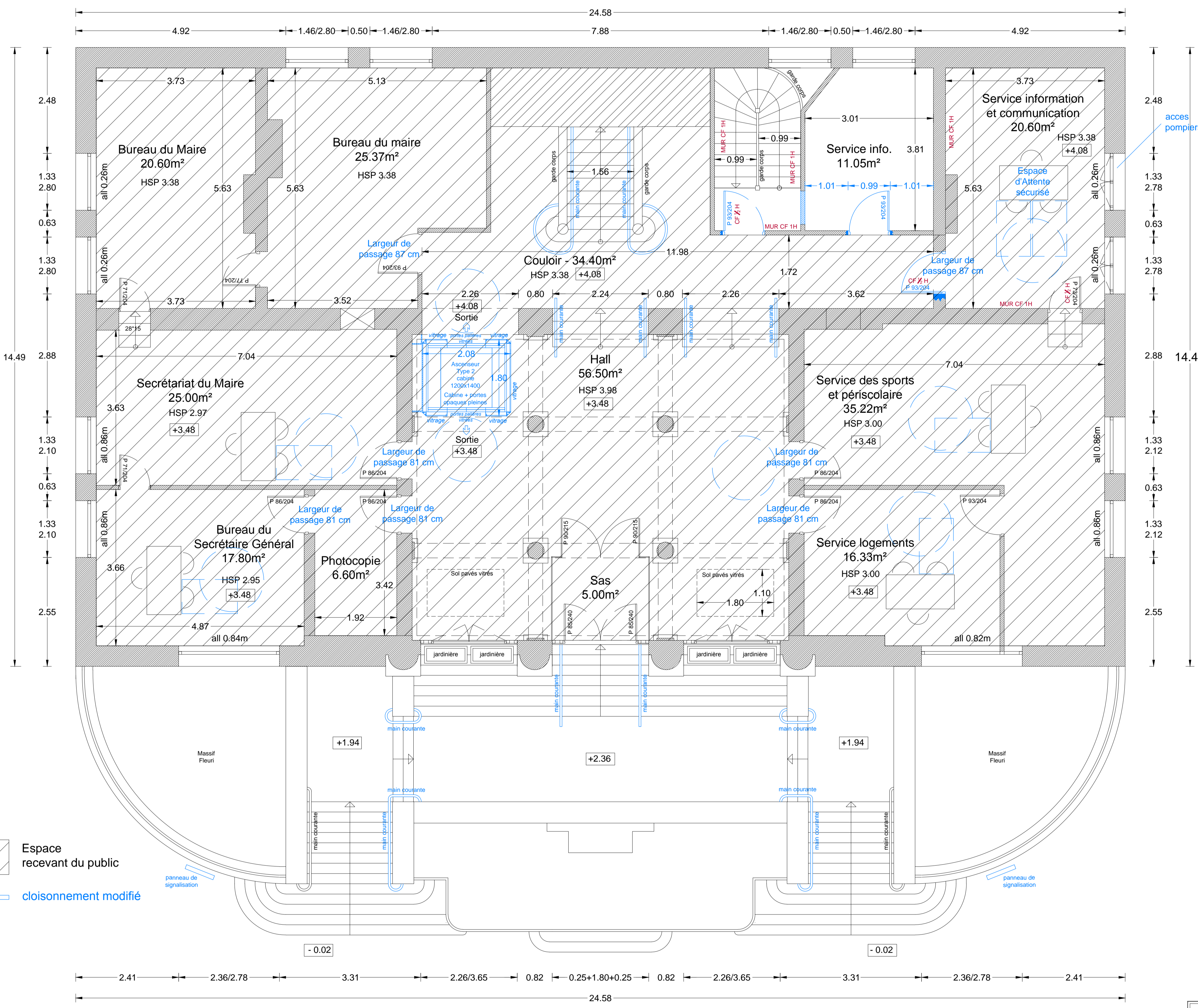
PLAN R+1 ECH : 1/50
